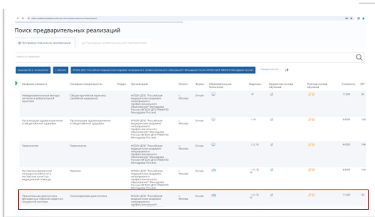
Рисунок 4 – выбор программы
