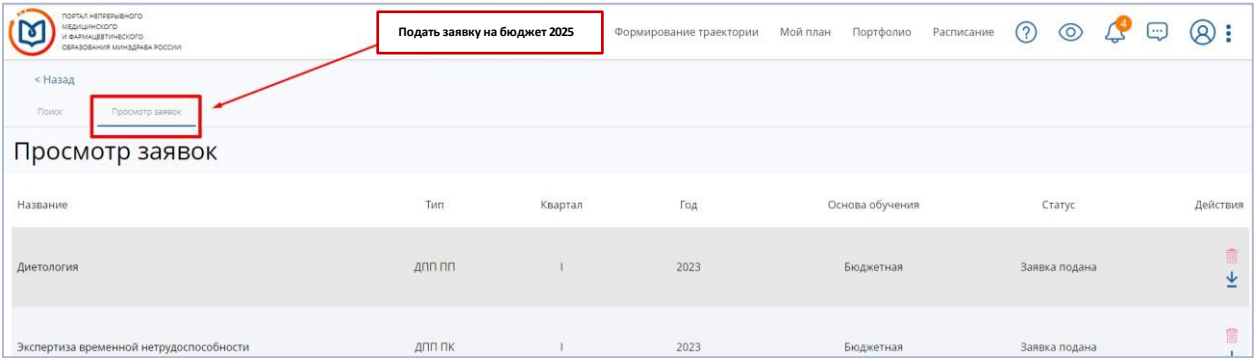
Рисунок 8 – Просмотр заявок
